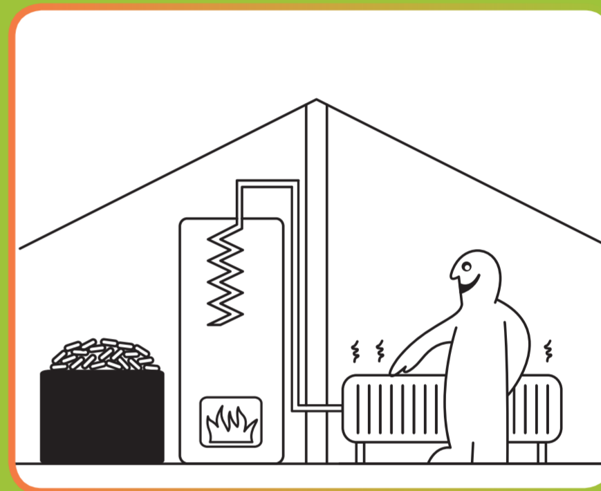
Pelletketel
